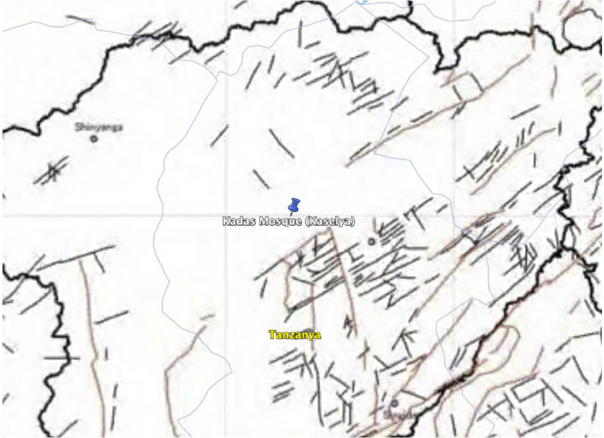
Şekil 4-ÇALIŞMA SAHASI VE CİVARINDAKİ FAYLAR VE KIRIK SİSTEMLERİ
