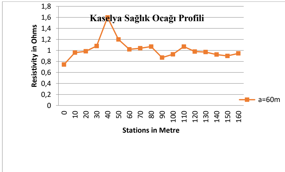
Şekil 8-Düşey Elektrik Eğrisi
